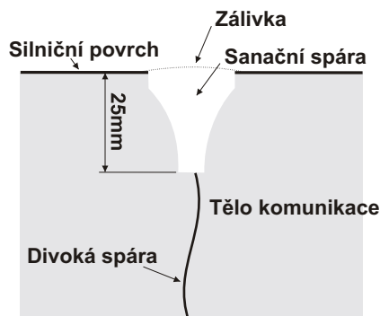
Profil komunikací
