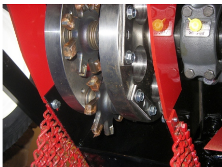
detail uložení frézovacích nástrojů
