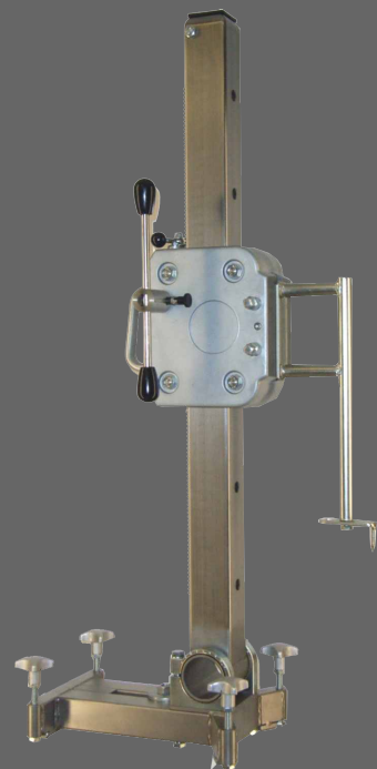
Středící adaptér
